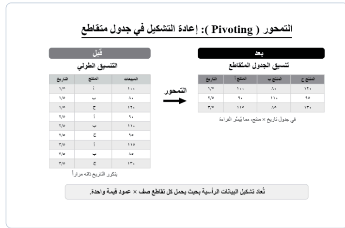
الشكل 5.2.2 – تحويل المحور: إعادة تشكيل البيانات ذات الصيغة الطويلة إلى جدول متقاطع
