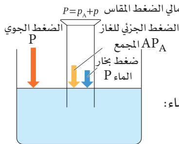
شكل 1.6.1 قياس الضغط الجوي
