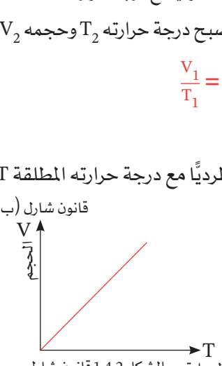
الشكل 1.4.2: قانون شارل
