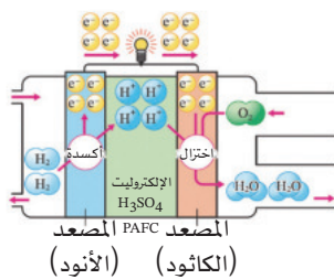
الشكل 2.4.2 خلية الوقود
