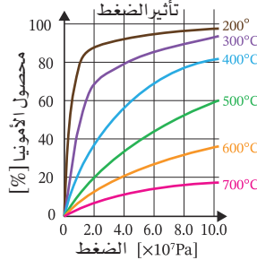
شكل 2.10.4 تأثير تخليق الأمونيا
