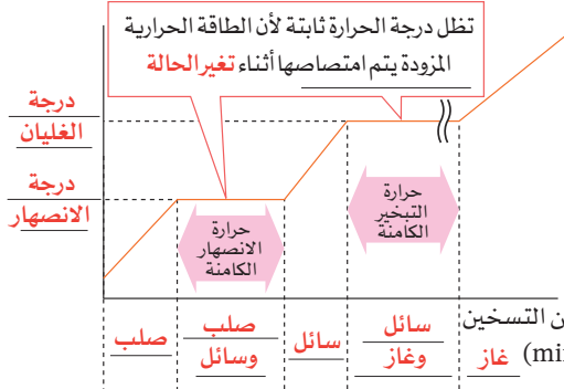
شكل 1.1.1 العلاقة بين تغير درجة الحرارة والحالة الفيزيائية للمادة
