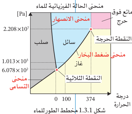
شكل 1.3.1 مخطط الطور للماء
